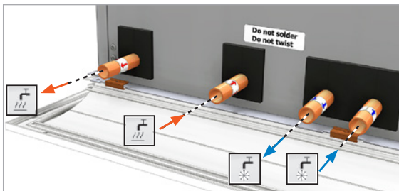
I-60: 4-rørs batteri (plus funktion).
