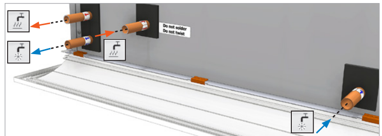
I-120: 4-rørs batteri (plus funktion).
