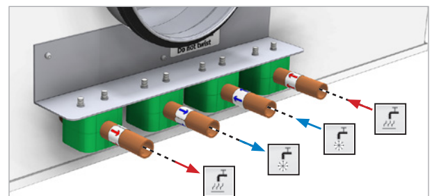
F model: 4-rørs batteri (plus funktion).
