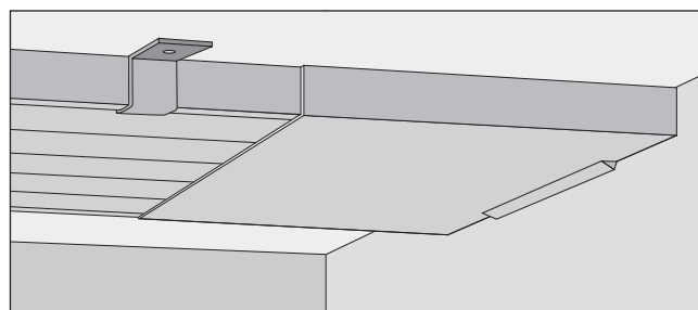
Figur 1. Atrium med tilslutningskappe. (ATR-CW).
