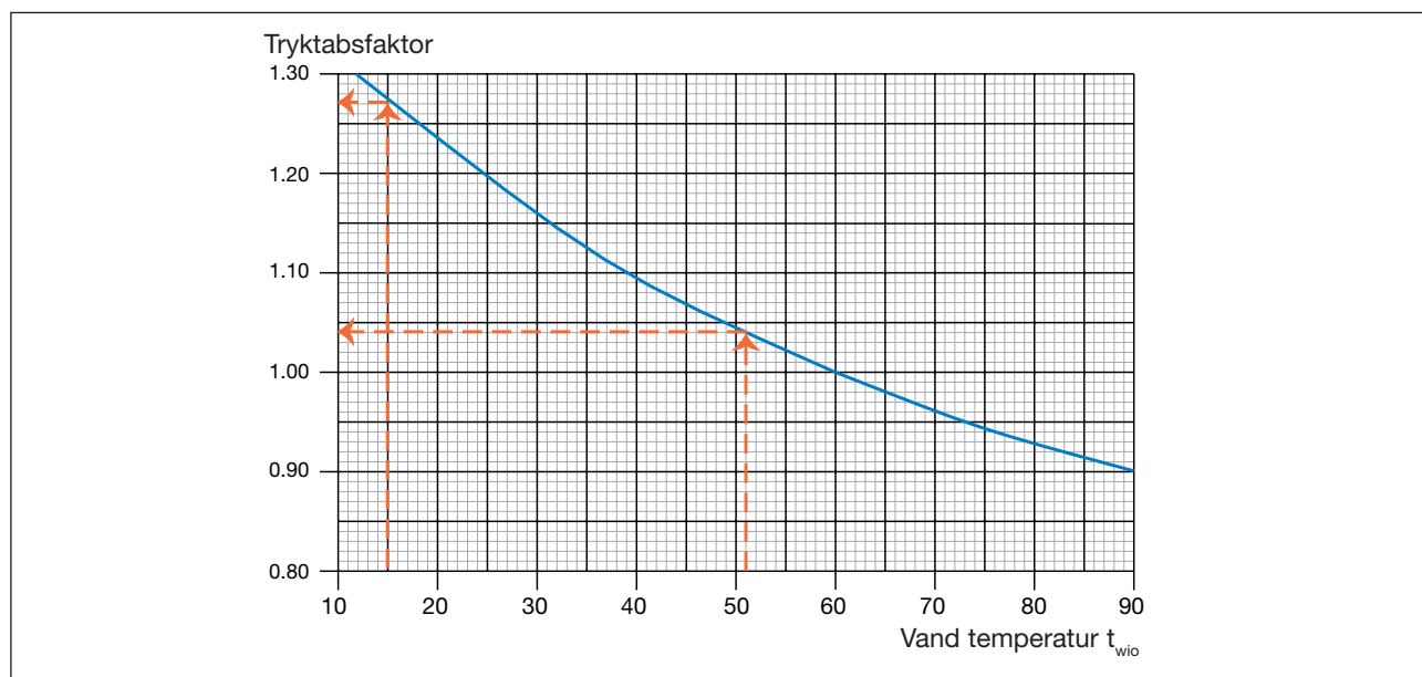
Diagram 7. Temperaturkorrigeret tryktabsfaktor.
